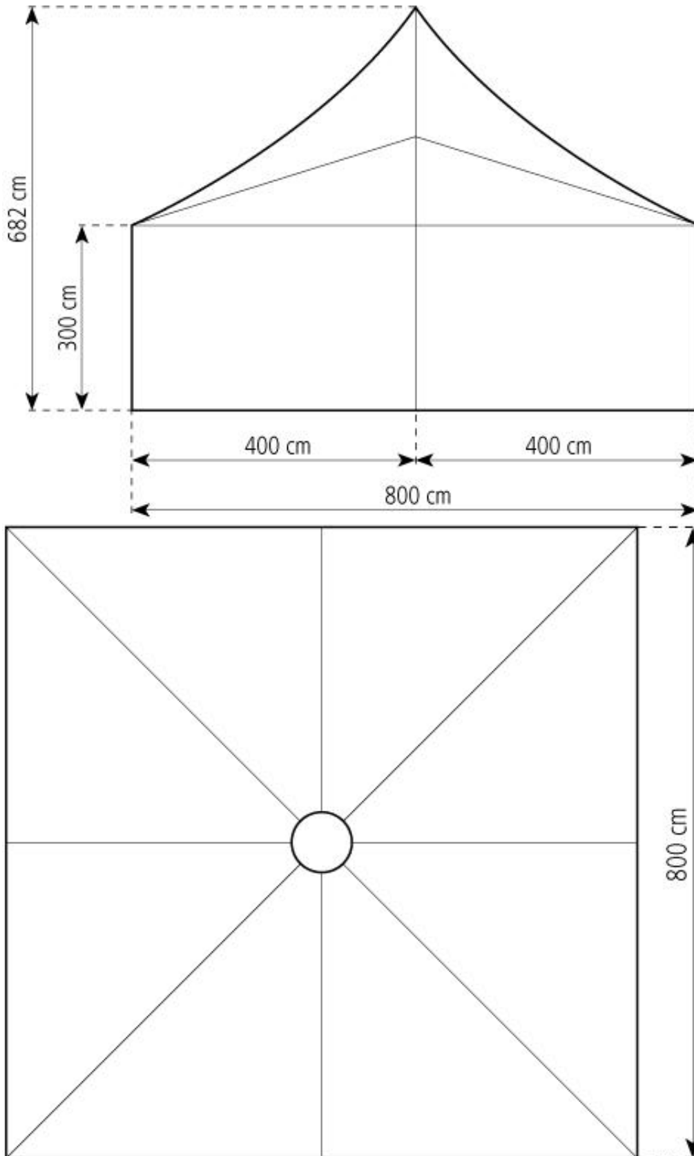
篷房俯视图与侧视图
