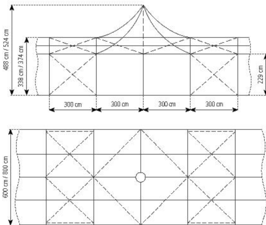
篷房俯视图与侧视图
