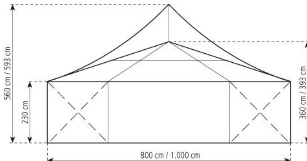
篷房俯视图与侧视图
