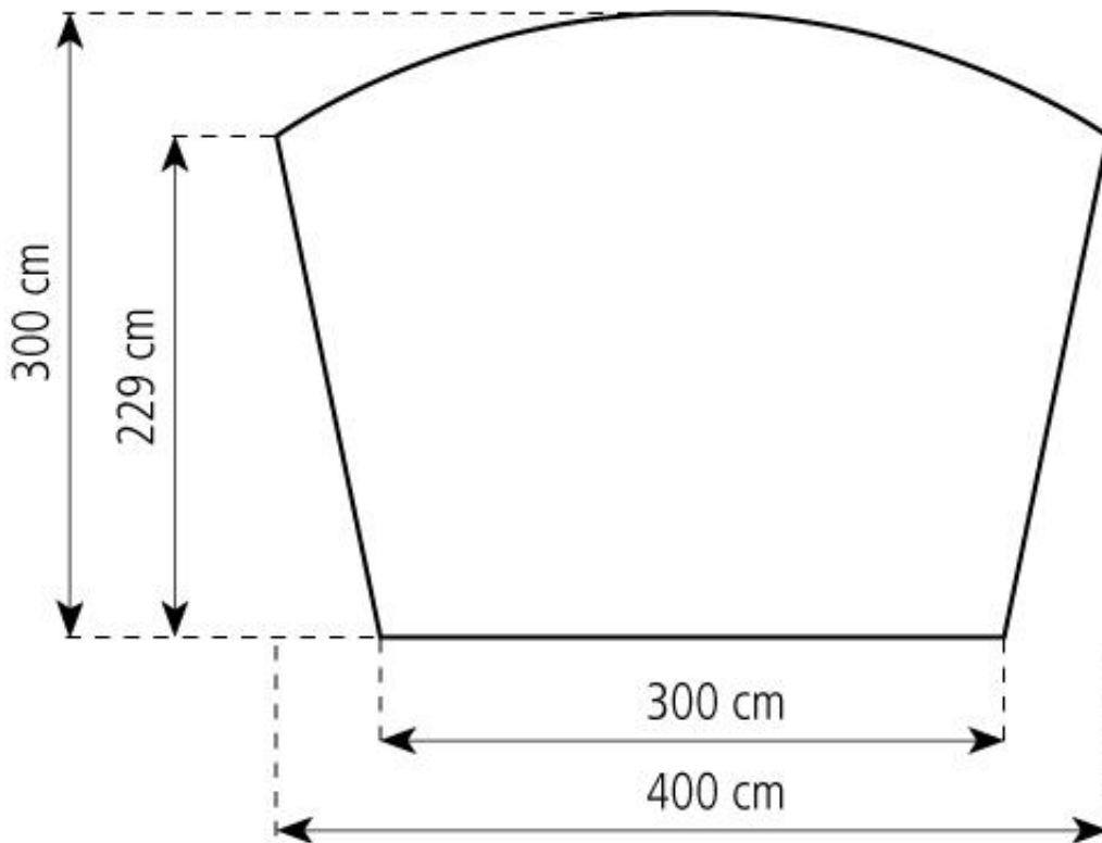
篷房俯视图与侧视图
