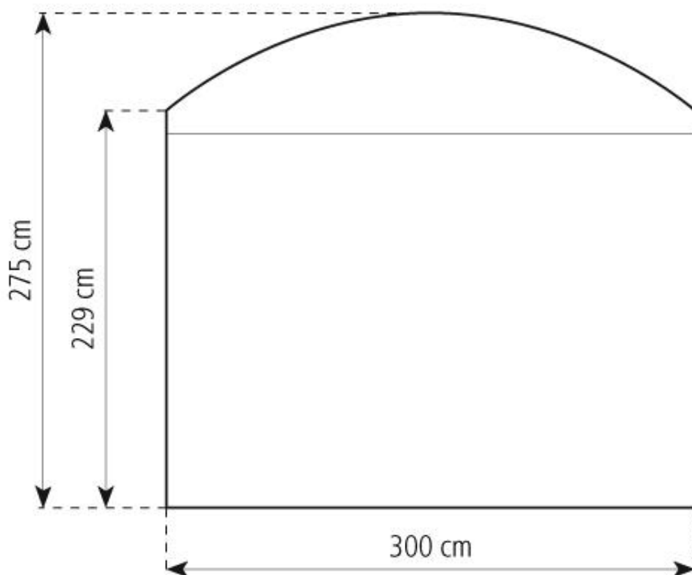
篷房俯视图与侧视图
