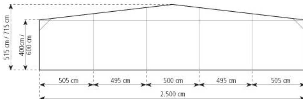
篷房俯视图与侧视图
