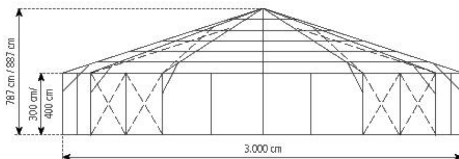
篷房俯视图与侧视图
