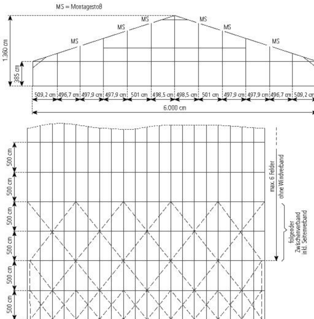
篷房俯视图与侧视图
